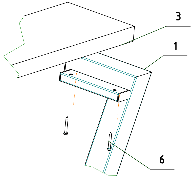
B ( 1 : 5 )
